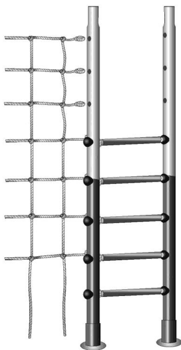
Рис.2 Сборка лестницы
